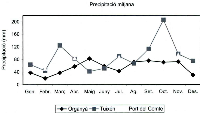
FIGURA 5. Precipitació mitjana (mm) mensual per a Organyà, Tuixén i Port del Comte.
