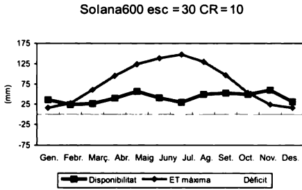
Gràfica del balanç hídric per a Solana600
