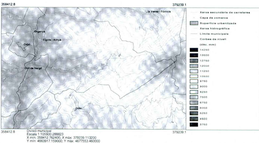
FIGURA 6. Precipitació anual (mm × any -1 ) per a la zona d'estudi. Font: Atlas climàtic digital de Catalunya .
