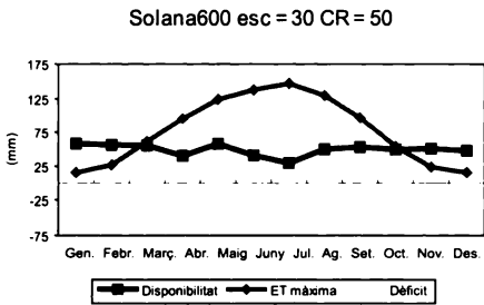
FIGURA 12.1. Distribució de la disponibilitat, l'evapotranspiració màxima i el dèficit existent en els diferents subescenaris: Solana600, Obaga1200.
