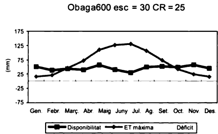
Gràfica del balanç hídric per a Obaga600
