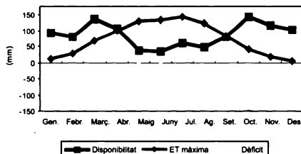
FIGURA 12.2. Distribució de la disponibilitat, l'evapotranspiració màxima i el déficit existent en els diferents subescenaris: Solana1200, Obaga1200.
